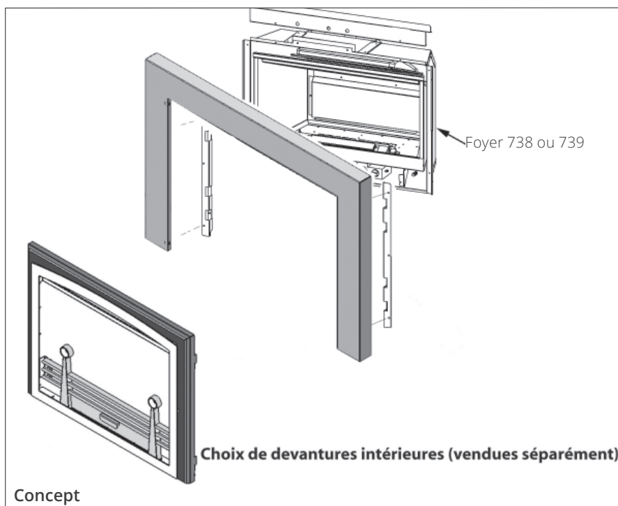
Bordure angulaire 756 montrée avec la Porte simple FenderFire optionnelle (D'autres devantures sont disponibles)
